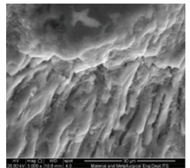
Hasil Uji SEM kelembaban 60%
