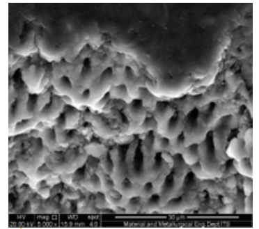
Hasil Uji SEM kelembaban 40%
